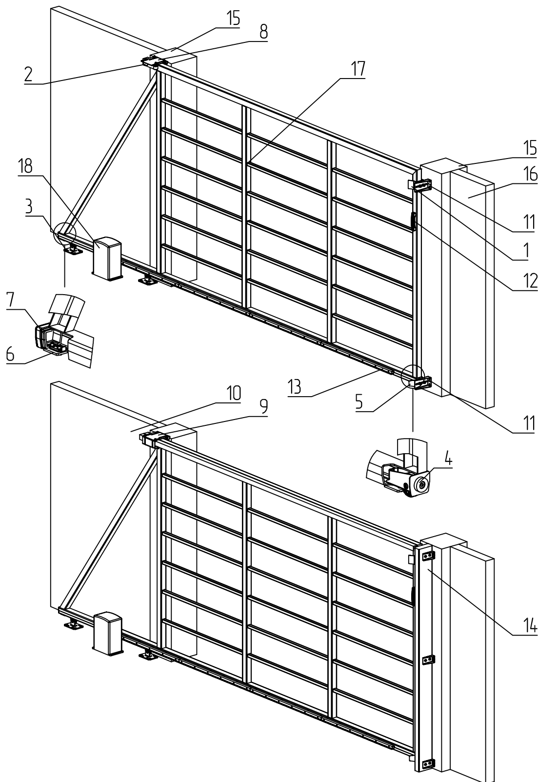
Рисунок 1 - Откатные самонесущие ворота, открытие: влево
