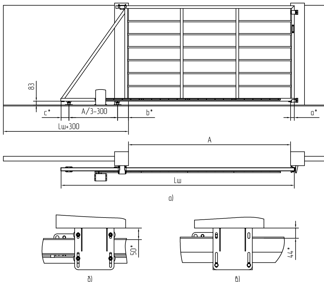
Рисунок 2 – Схема откатных самонесущих ворот, открытие: влево
